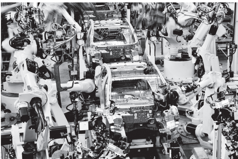
▲宁波杭州湾新区吉利汽车装配车间
